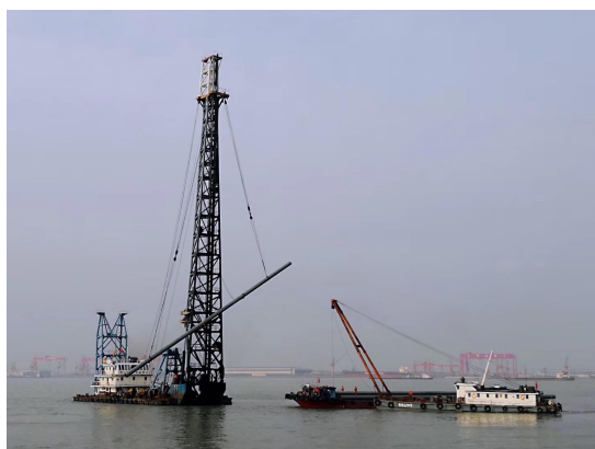
取水头部保护桩正在施工
